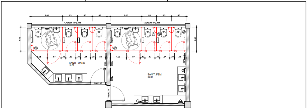
PLANTA BAIXA - SANITÁRIOS SEGUNDO PAV. 1/50
